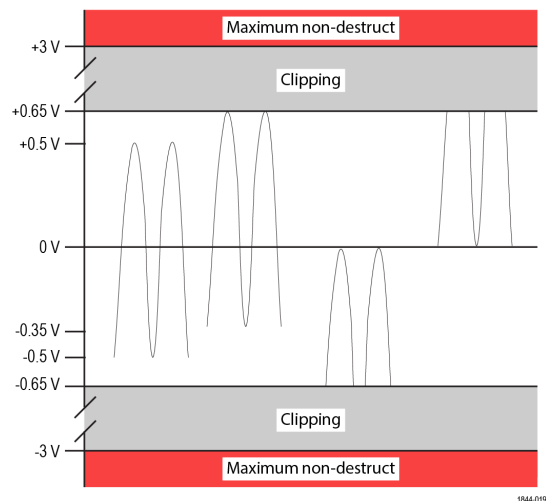
Plage de tension d'entrée différentielle
