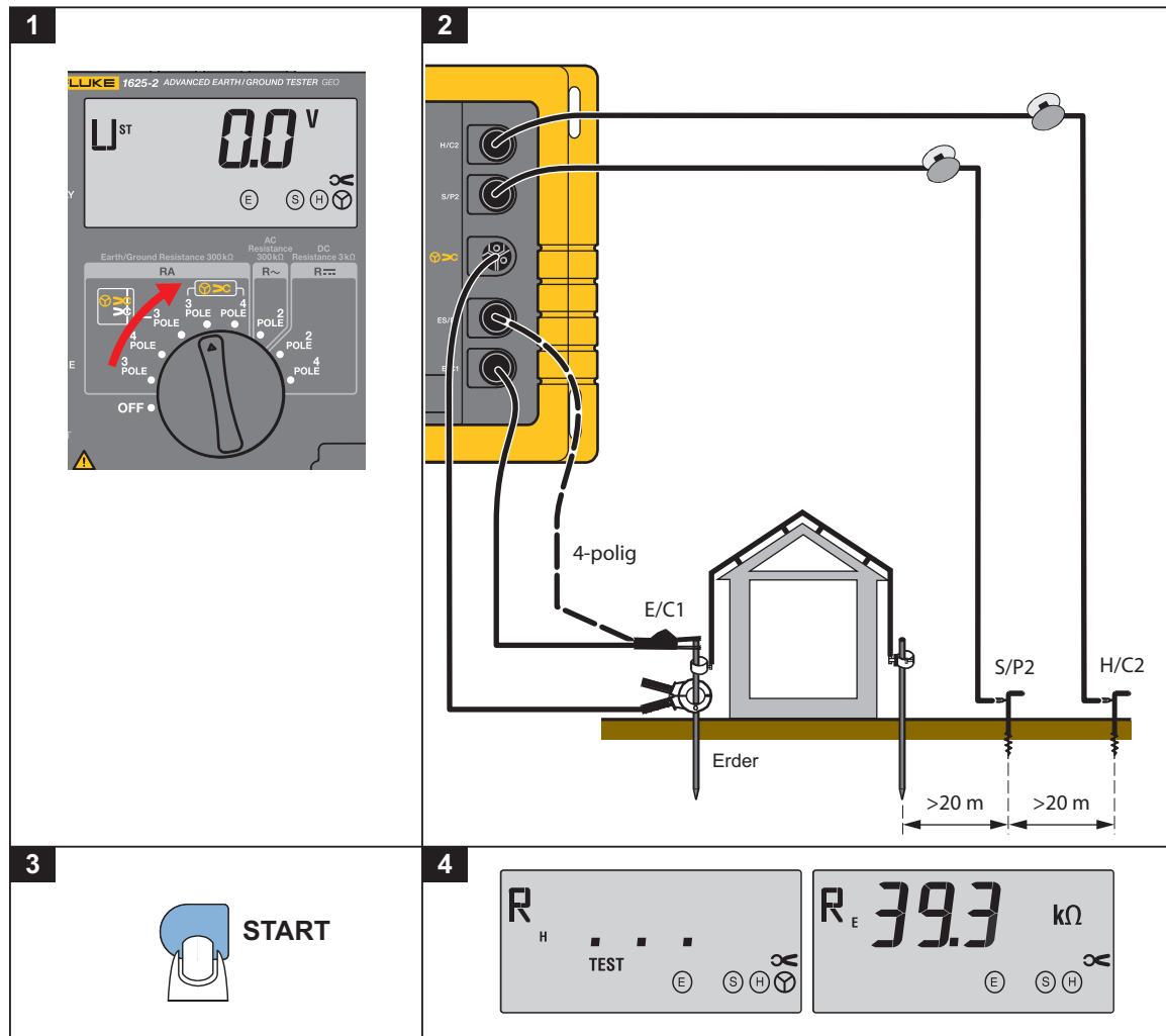
Abbildung 6. Einzelerderwiderstandsmessung 3-polig/4-polig
